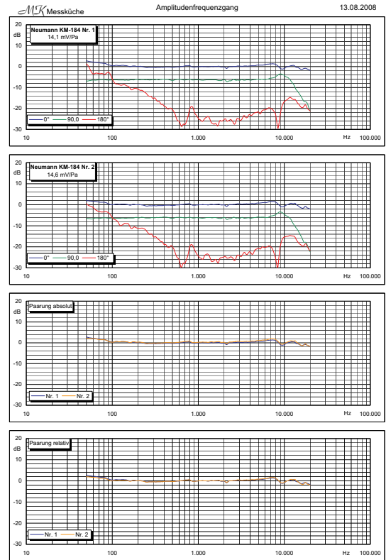
Gemessene Frequenzgänge des Testsiegers Neumann KM-184: Bis auf eine leichte Welligkeit im Hochtonbereich verlaufen die 0-Grad-Frequenzgänge (blaue Linien) vorbildlich linear. Der Bassanstieg unterhalb 100 Hz dürfte auf den Nahbesprechungseffekt zurückzuführen sein, die leichte Senke bei 2100 Hz zeigt den Einfluss (Reflexion) der Mikroklammer. Die grünen Linien (seitliche Schalleinwirkung 90 Grad) verlaufen über einen weiten Bereich knapp unterhalb -6 dB, die roten unterhalb -20 dB, so dass hier die Mikrofone die Nierencharakteristik sauber einhalten.
