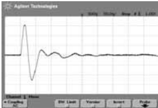
Die von uns aufgenommene Impulsantwort des zweitplatzierten Shure KSM-137: Zwei saubere Halbwellen markieren das Hin- und Rückschwingen der Membran als Reaktion auf den einmaligen Schallimpuls, während die Nachschwinger in Auslenkung und Anzahl vernachlässigbar gering ausfallen.
